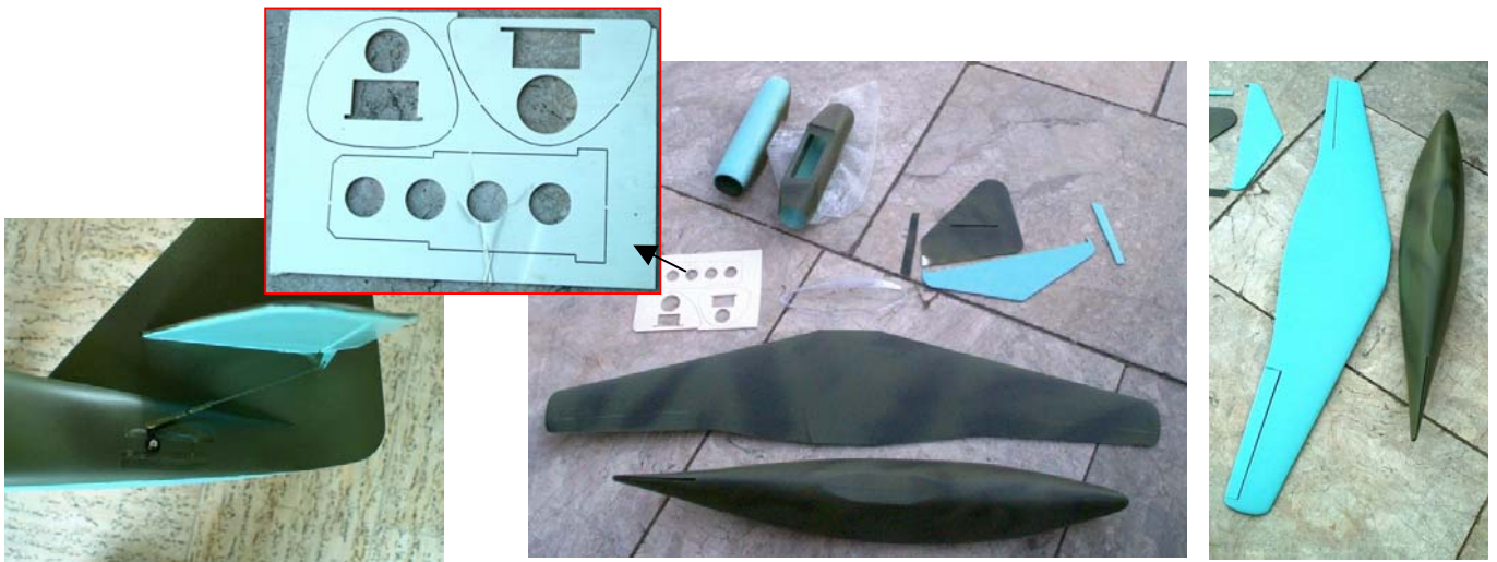
Unten: Lieferumfang der in Scale-Farben lackierten Voll-Gfk-Version. Das vergrößerte Bild zeigt die beiden Rumpfspanten, die vor der Fläche im Rumpf eingearzt werden und darunter die Akkuschublade, die eingeschoben wird und zum Aufladen durch die Flächenöffnung herausziehbar ist!
