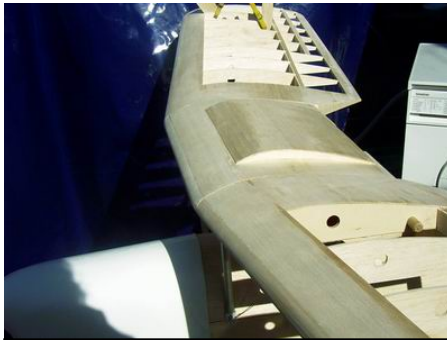
Obere Tragfläche einteilig
